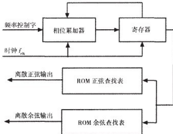
图3 NCO结构图
